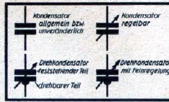
Man kann in Schaltbildern nicht Kondensatoren in ihrer wirklichen Form zeichnen. Deshalb verwendet man für die einzelnen Kondensatorarten diese Schaltzeichen.
